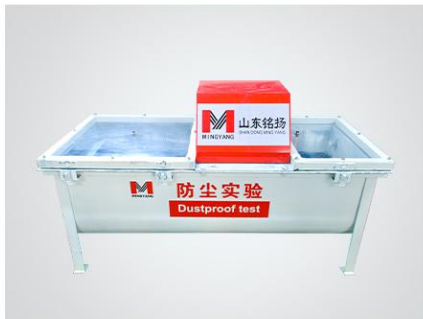
Dustproof Tester 防尘试验机
