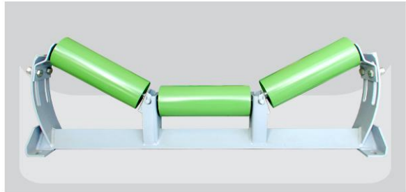
Transition Idler 可调角度托辊组
