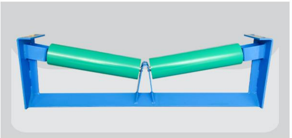
V-return Idler V型托辊组
